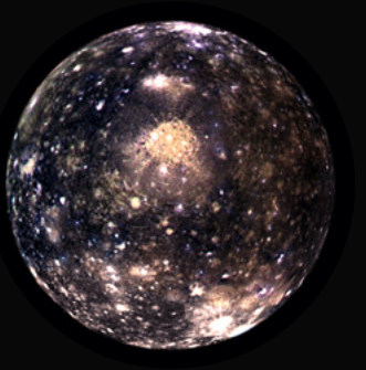
Callisto
