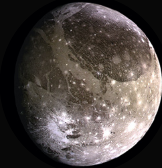
Ganymède
